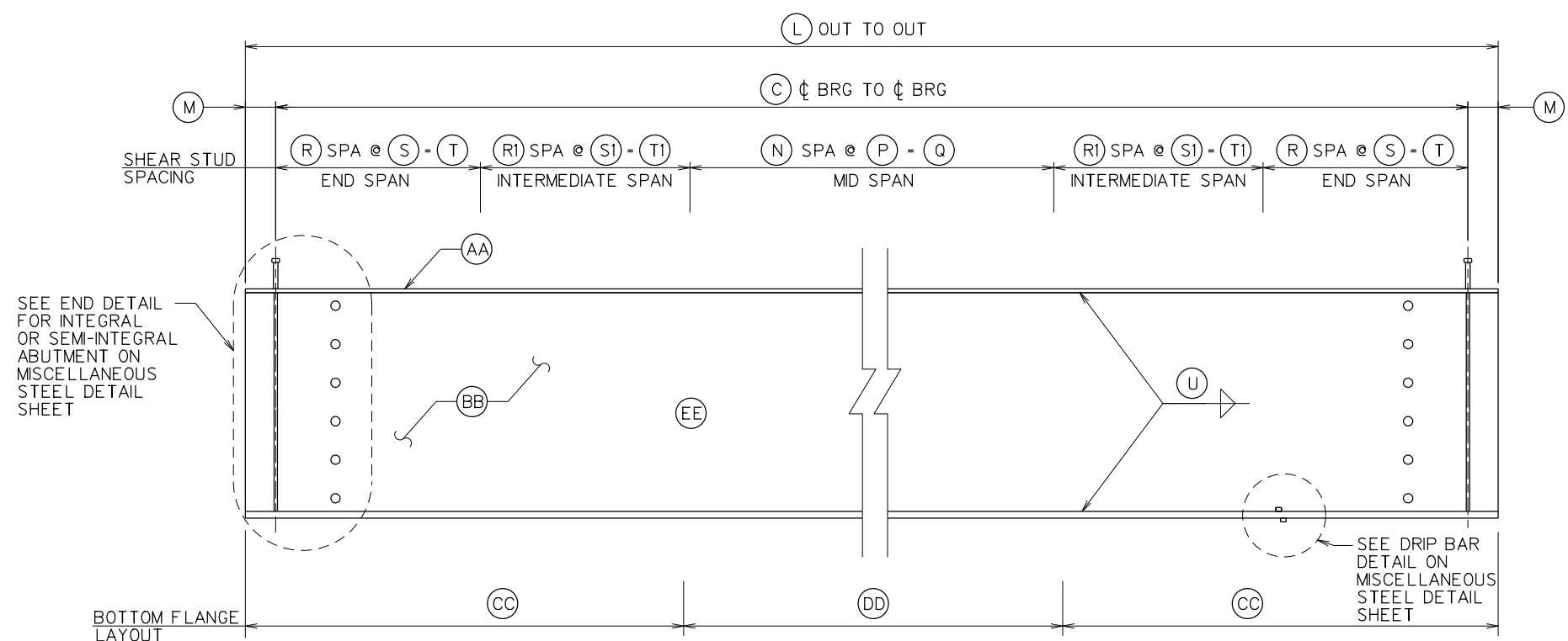
ELEVATION
