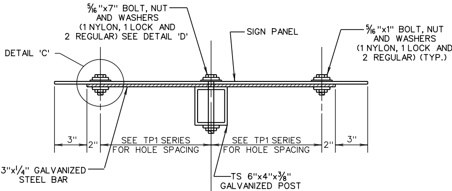
DETAIL 'B' - TOP VIEW N.T.S.
