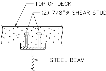
SHEAR STUD DETAIL
